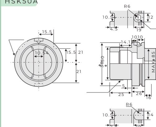
HSK50A
