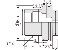
HSK50E
